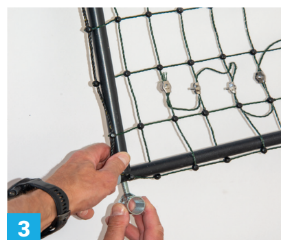
3 Mocowanie przegrody za pomocą ele- mentu zawieszania A válaszfal rögzítése függesztőelem segítségével
