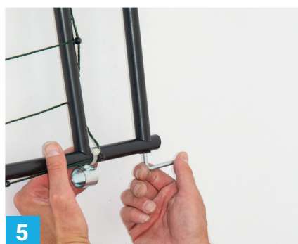
5 Mocowanie przegrody za pomocą śruby A válaszfal rögzítése csavarral
